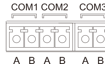
图 4.2-1 EzLogger Pro的COM1、COM2、COM3口示意图
