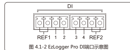
图 4.1-2 EzLogger Pro DI端口示意图
