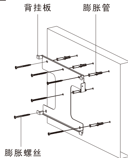
背挂板安装
