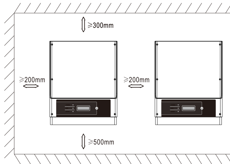
安装距离
